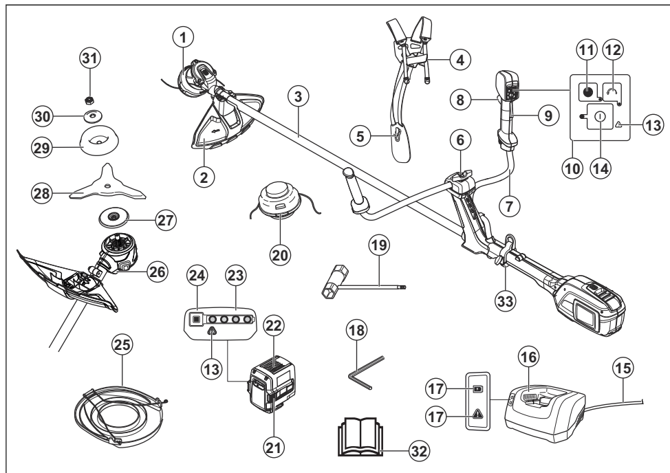
1. Trimmerhode
